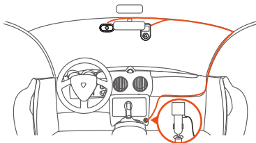
DMS镜头安装和布线参考图
